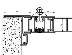
TELAIO CON COMPENSATORE A Z COD: BR003
