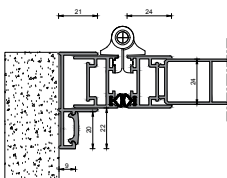
TELAIO CON COMPENSATORE A L COD: BR002
