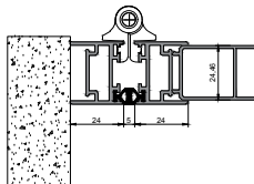
TELAIO SENZA COMPENSATORE COD: BR001
